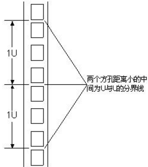
图 9-5 机柜导槽 U 与 U 的间距区分示意图
