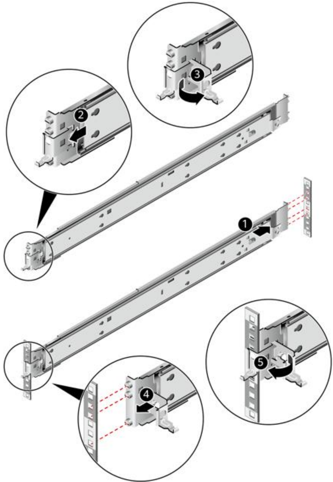
图 9-11 安装抱轨
