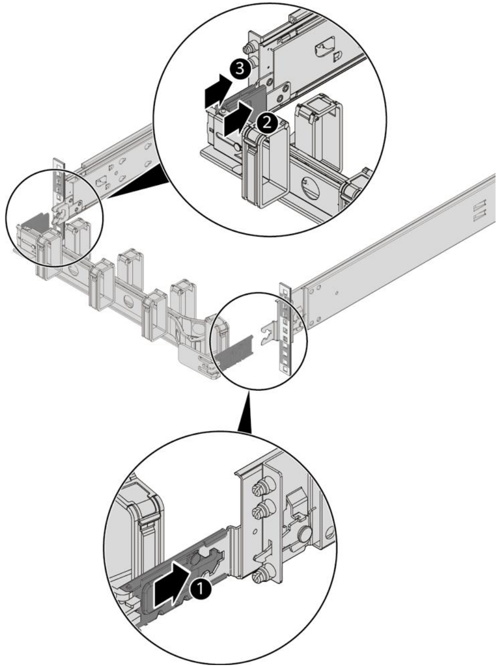
图 9-17 安装理线架
