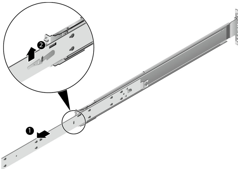
图 9-12 抽出内轨
