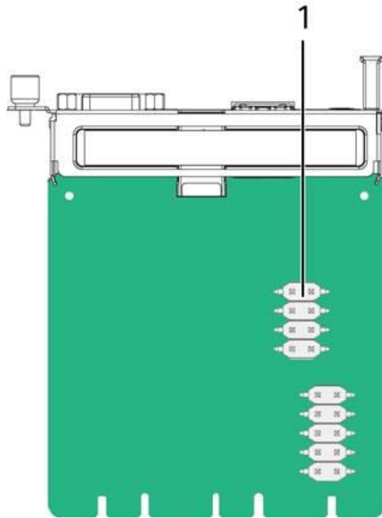
图 6-28 BMC 插卡
