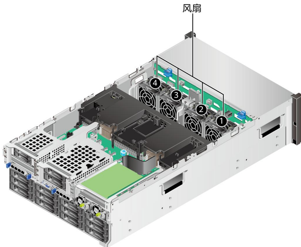
图 6-7 风扇位置图
