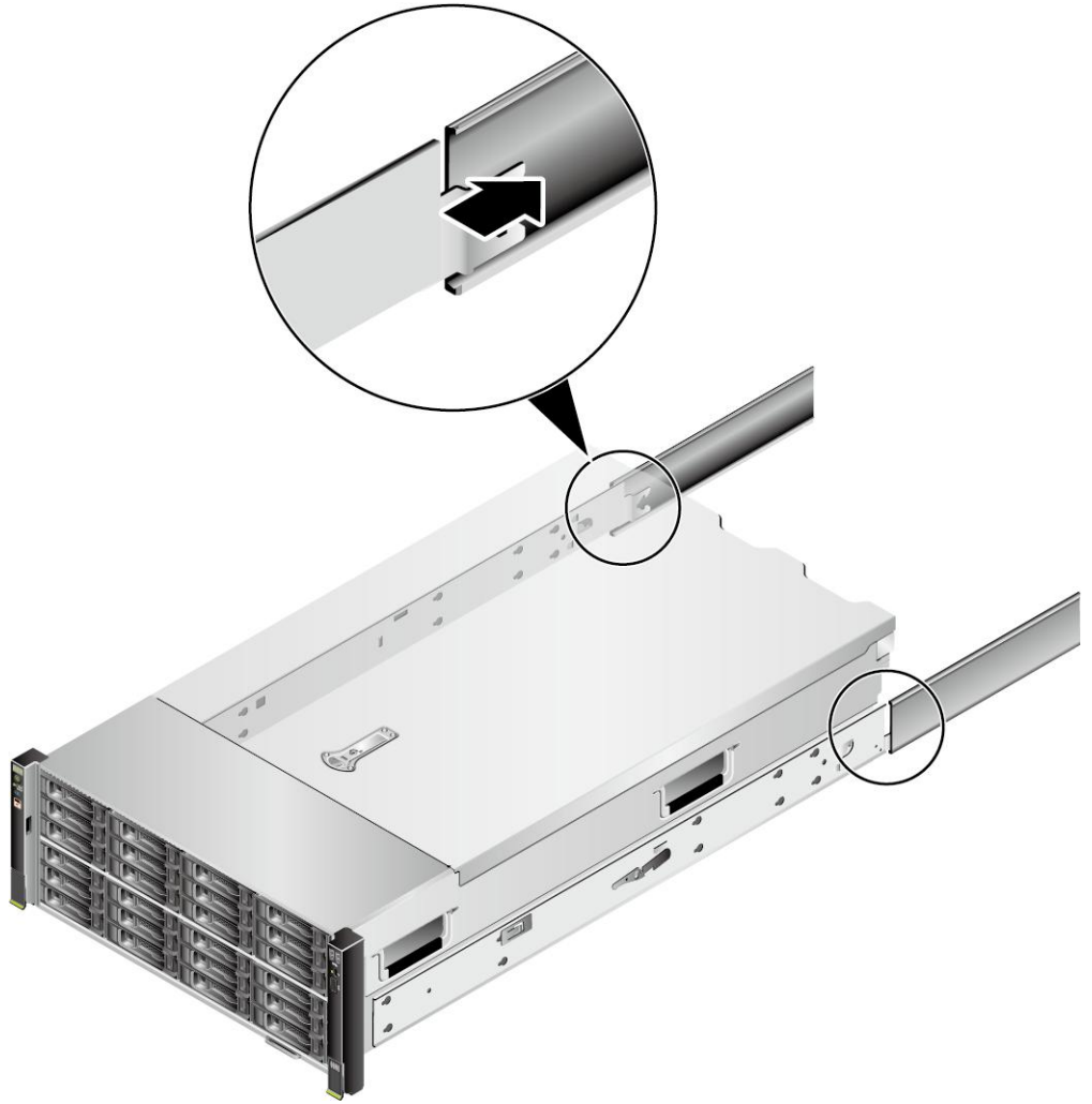
图 9-14 安装服务器
