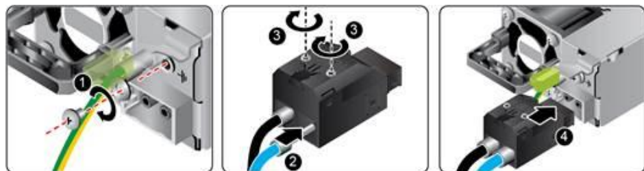
图 9-28 连接电源线缆（2000W 电源模块）
