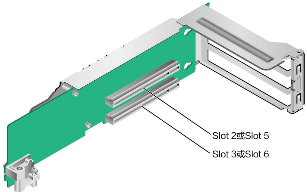
图 6-21 2*x8 Riser 卡
