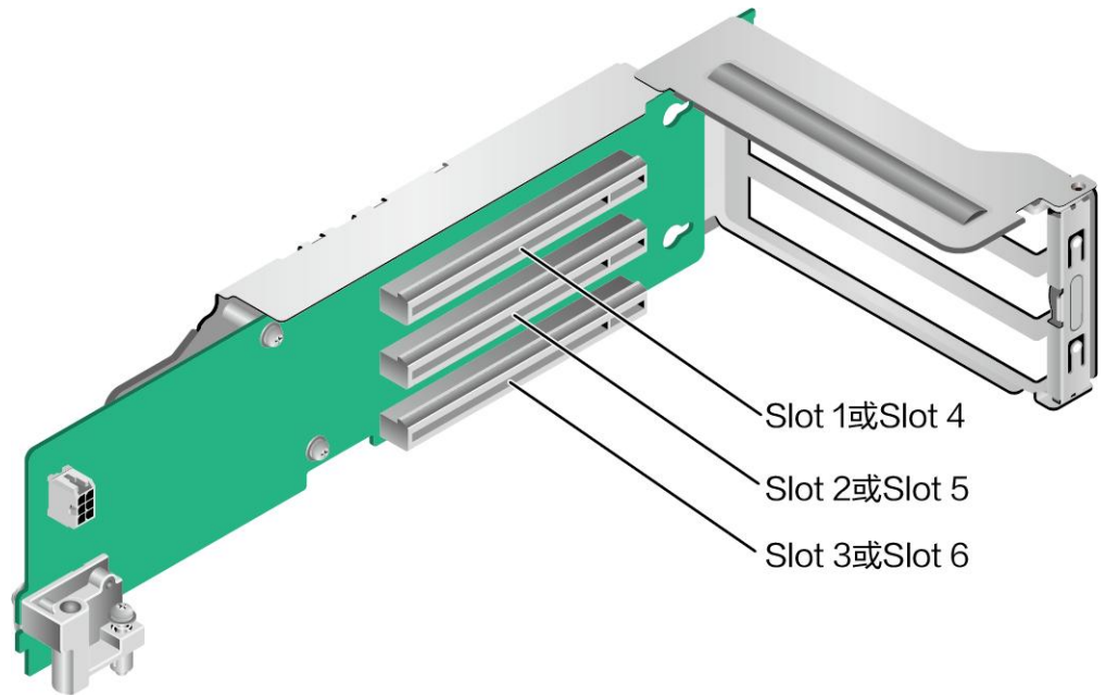
图 6-20 3*x8 Riser 卡
