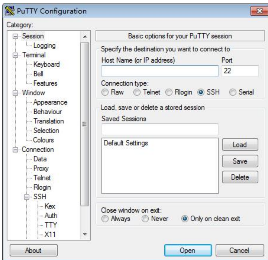
图 11-14 PuTTY Configuration
