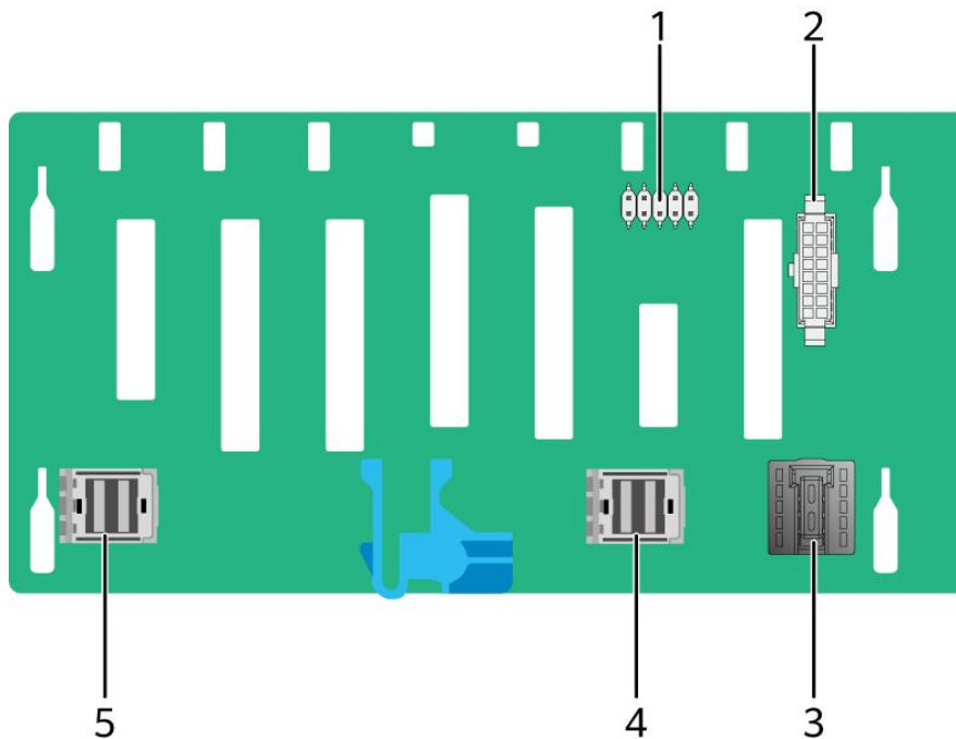
图 5-20 8x2.5 英寸硬盘 RAID 直通配置硬盘背板
