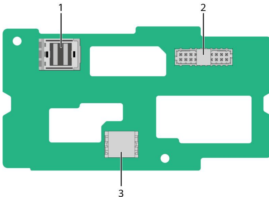
图 5-22 2x3.5 英寸后置硬盘背板
