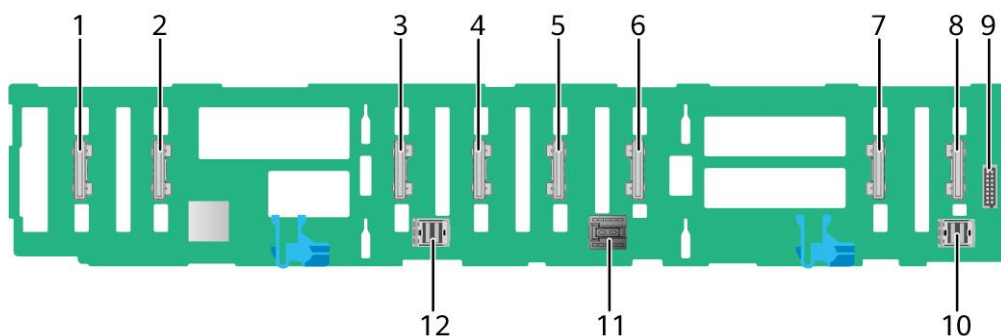
图 5-18 12x2.5 NVMe 硬盘配置硬盘背板
