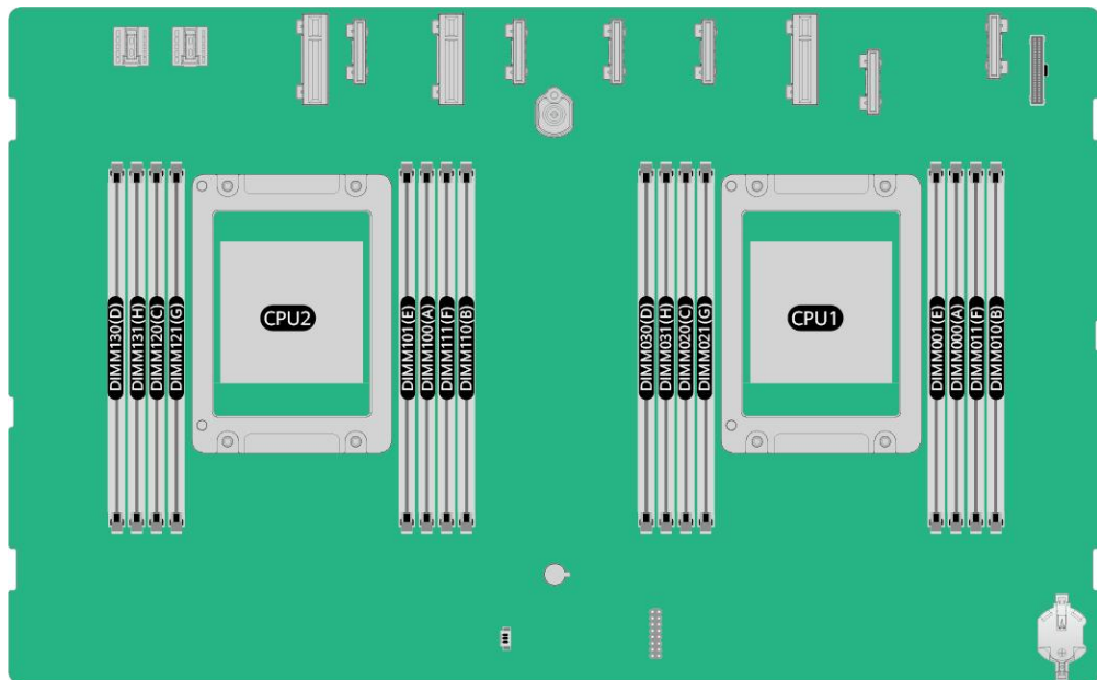
图 5-6 内存槽位编号
