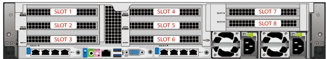
图 5-33 PCIe 插槽
