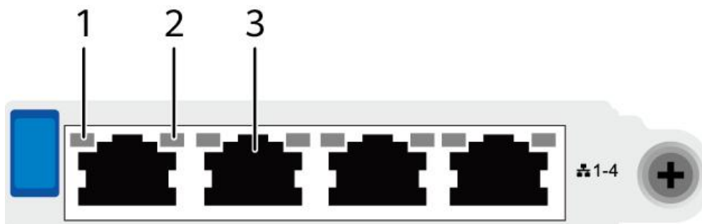
图 5-34 SF221Q (4xGE 电口)
