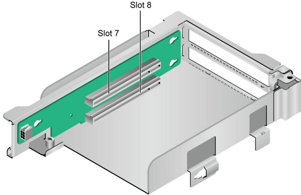
图 5-32 2*x8 Riser 卡
