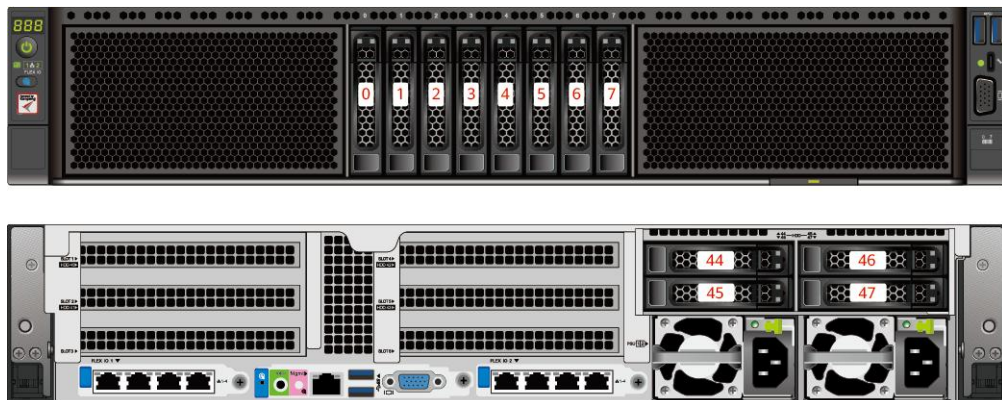
图 5-12 8x2.5 英寸硬盘 RAID 直通配置硬盘编号
