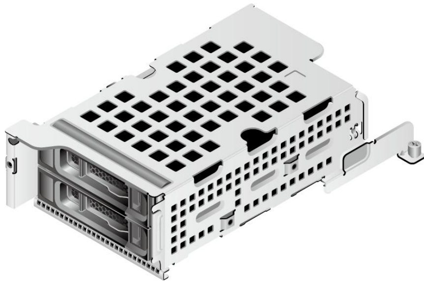
图 5-15 后置 2x3.5 英寸硬盘模组
