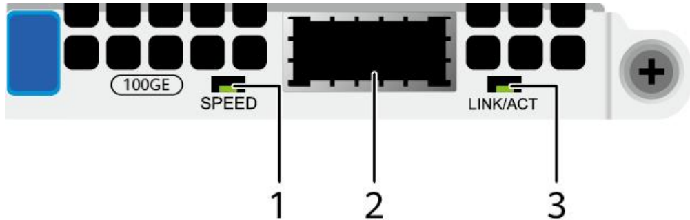
图 5-36 SF225S-H (1x100GE 光口)
