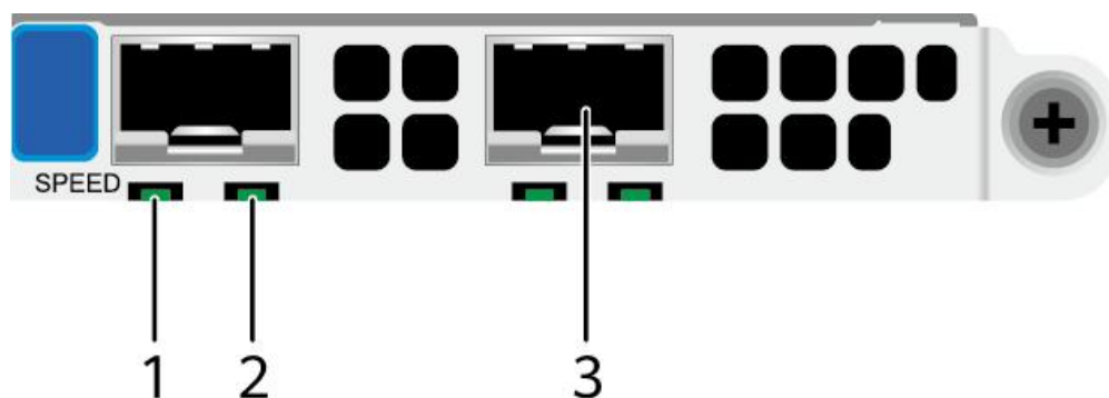
图 5-35 SF223D-H (2x25GE 光口)
