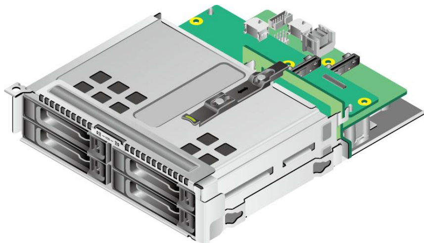
图 5-17 后置 4x2.5 英寸硬盘模组
