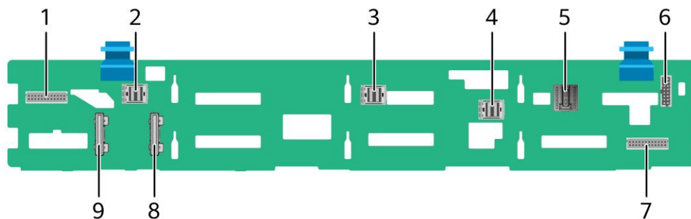
图 5-21 12x3.5 英寸硬盘 RAID 直通配置硬盘背板
