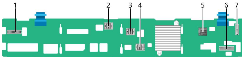
图 5-19 12x3.5 英寸硬盘 EXP 配置硬盘背板
