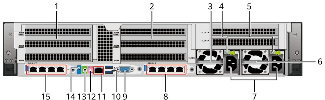
图 5-4 后面板
