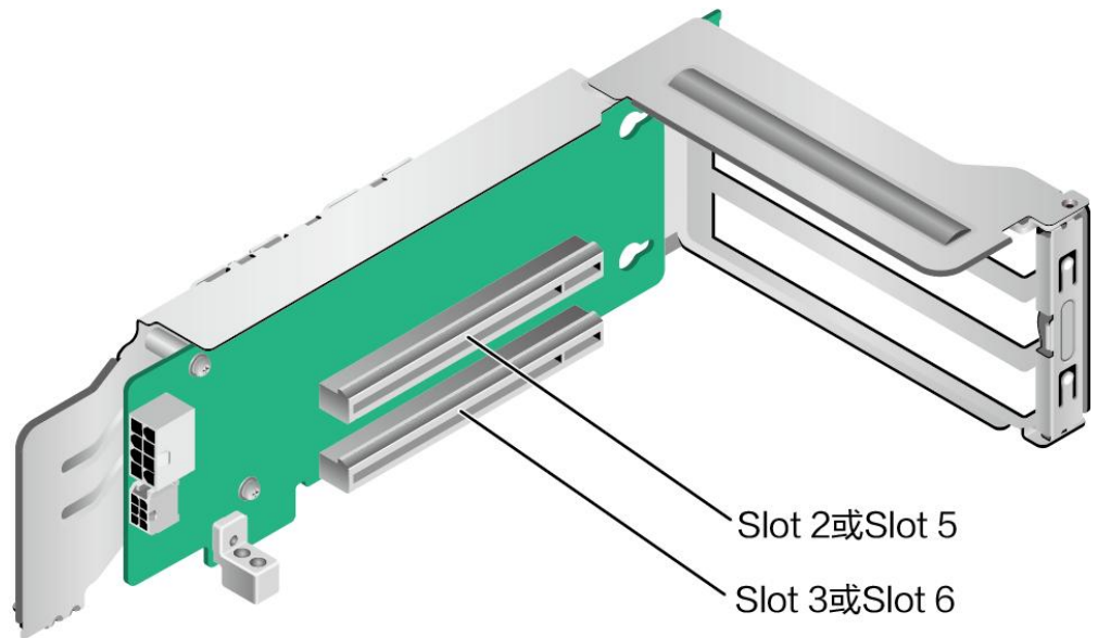
图 5-26 1*x16+ 1*x8 Riser 卡（正面）
