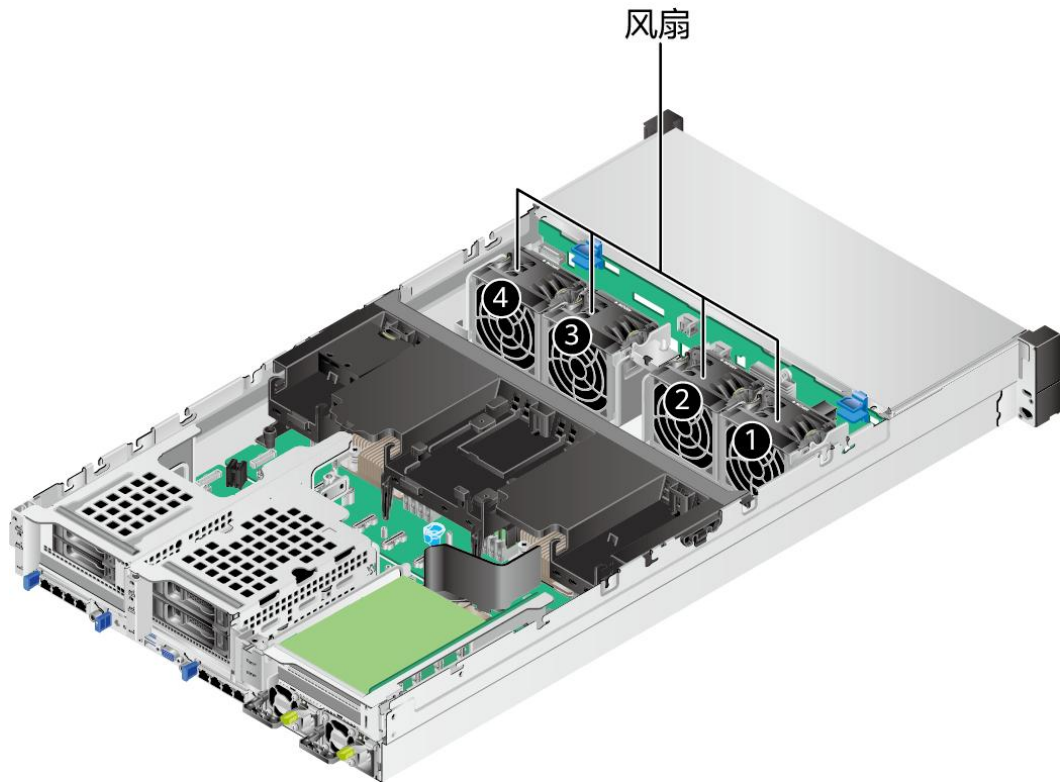
图 5-9 风扇位置图
