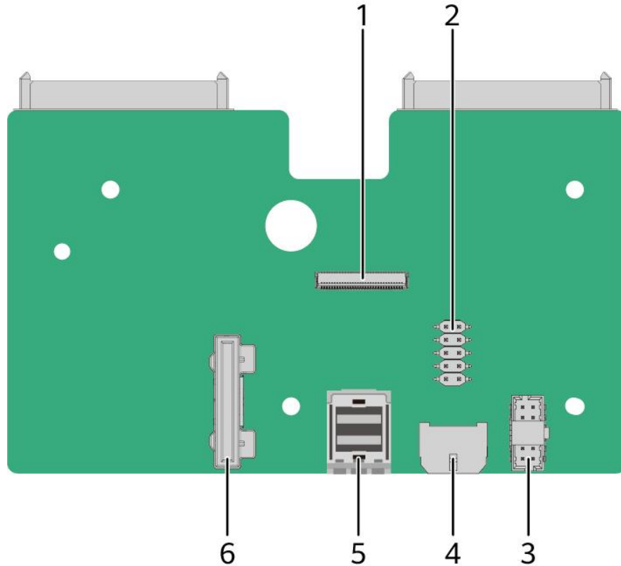
图 5-25 IO 模组 3 水平硬盘背板（下板）
