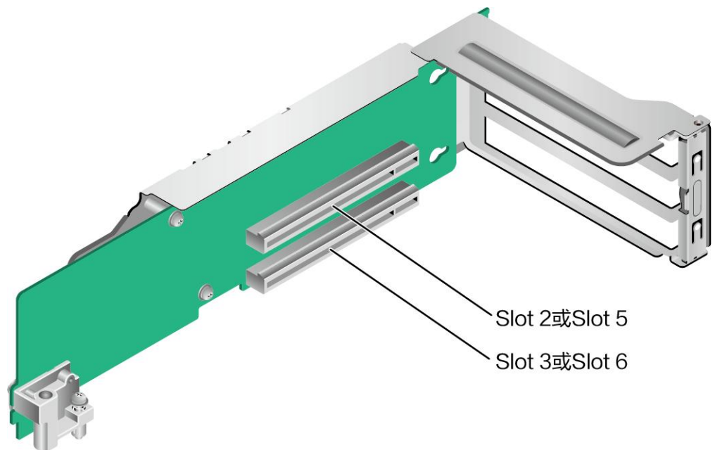
图 6-29 2*x8 Riser 卡
