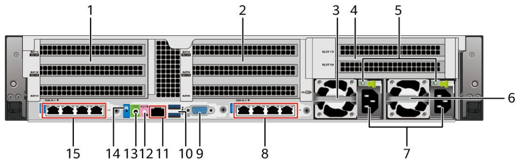
图 6-4 后面板
