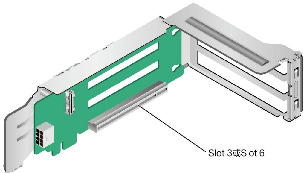
图 6-31 1*x8 Riser 卡
