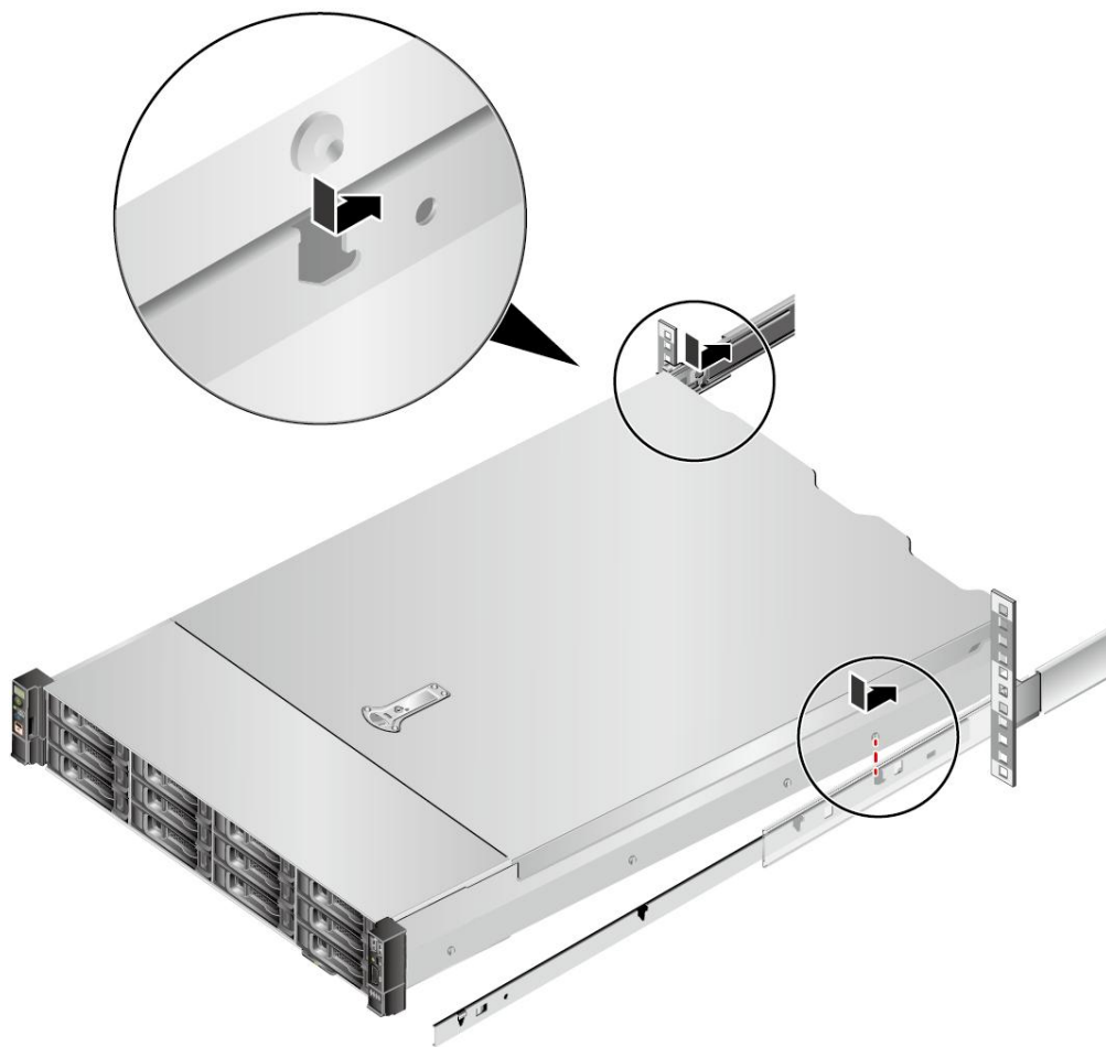
图 9-13 将服务器固定在内轨上 (1)
