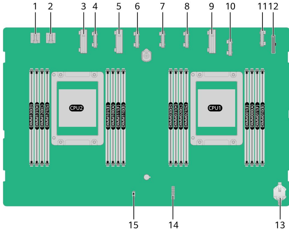
图 6-5 基础板接口
