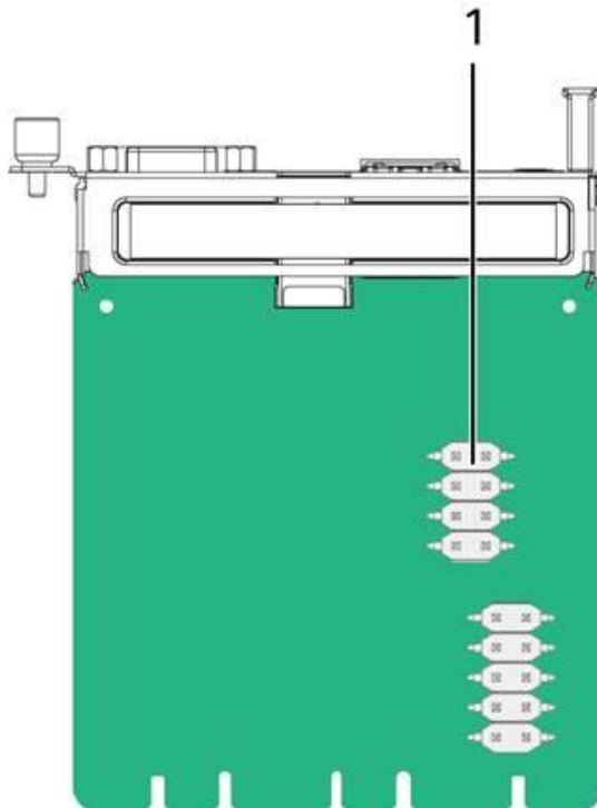
图 6-37 BMC 插卡
