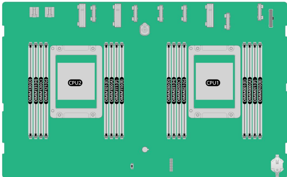
图 6-6 内存槽位编号
