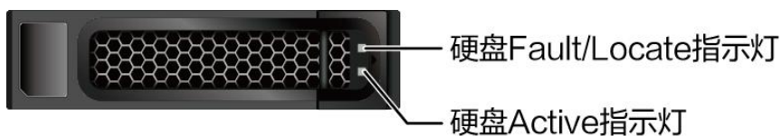
图 6-13 SAS/SATA 硬盘指示灯
