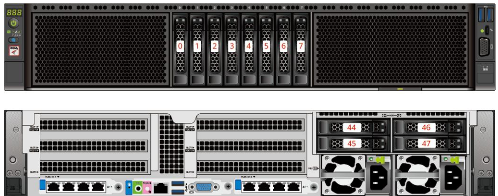
图 6-12 8x2.5 英寸硬盘 RAID 直通配置硬盘编号
