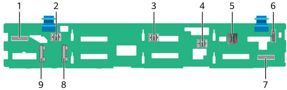
图 6-21 12x3.5 英寸硬盘 RAID 直通配置硬盘背板
