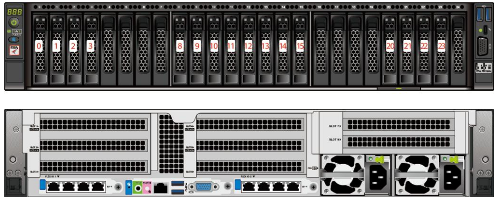
图 6-10 4x2.5 SAS/SATA+12x2.5 NVMe 硬盘配置硬盘编号
