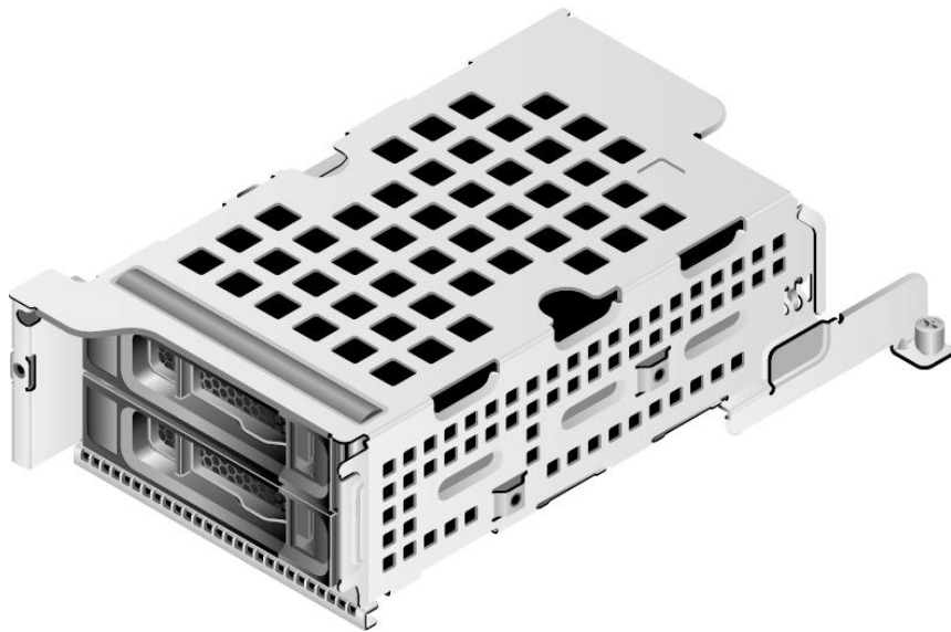
图 6-15 后置 2x3.5 英寸硬盘模组
