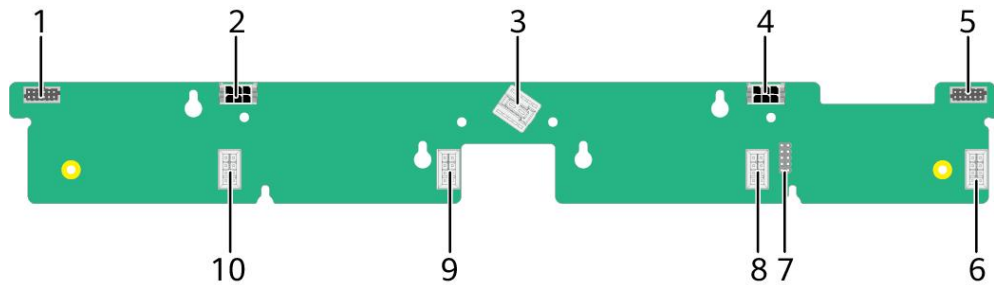
图 6-8 风扇板接口
