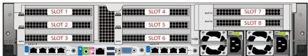
图 6-33 PCIe 插槽
