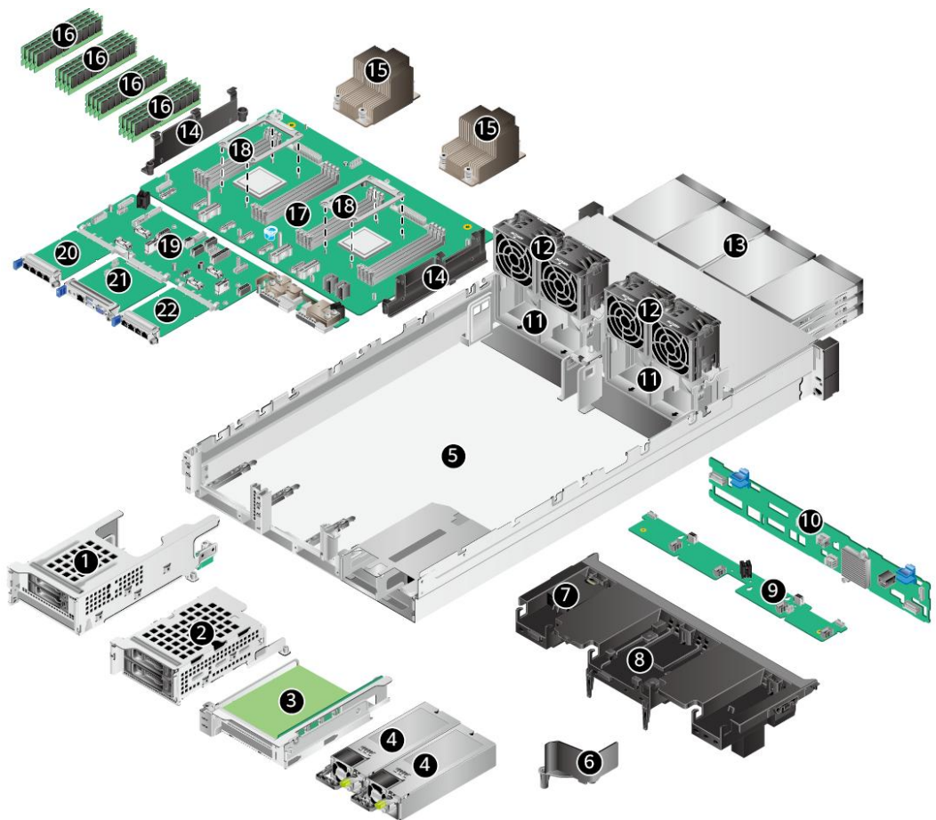
图 4-1 部件
