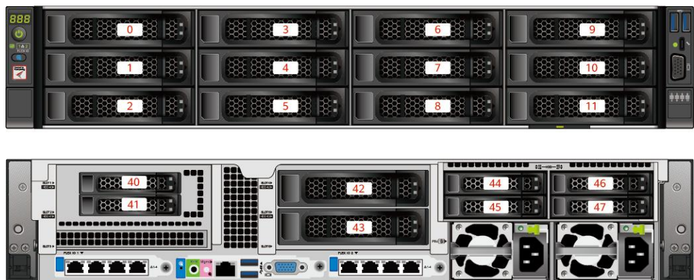
图 6-11 12x3.5 英寸硬盘配置硬盘编号
