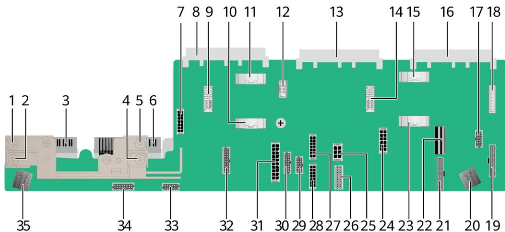
图 6-7 扩展板
