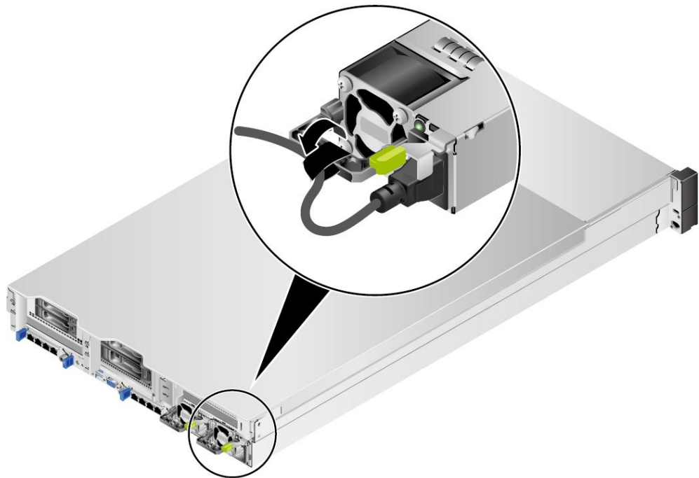
图 9-27 固定电源线缆
