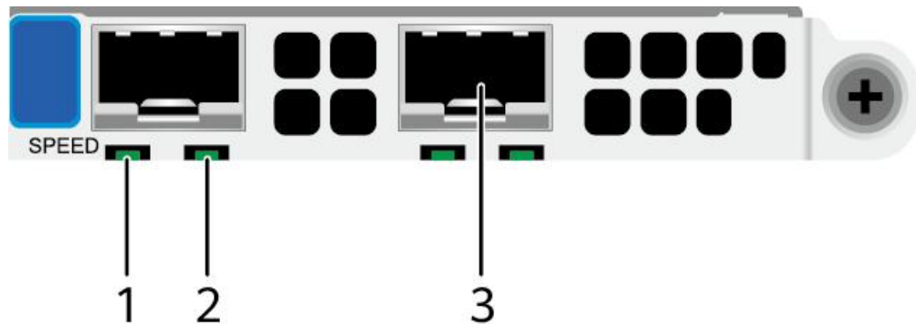
图 6-35 SF223D-H (2x25GE 光口)
