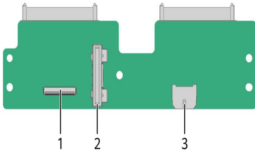
图 6-24 IO 模组 3 水平硬盘背板（上板）
