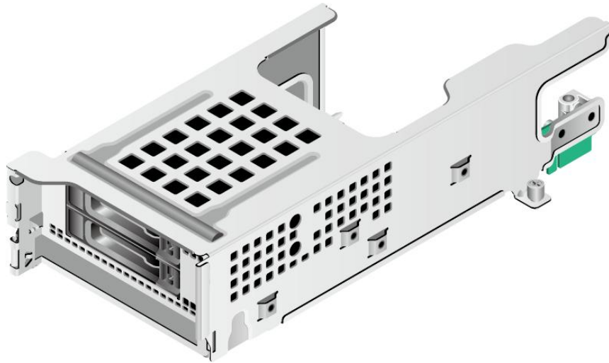
图 6-16 后置 2x2.5 英寸硬盘模组
