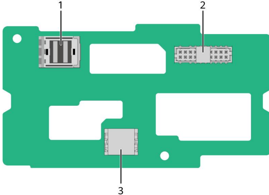
图 6-22 2x3.5 英寸后置硬盘背板
