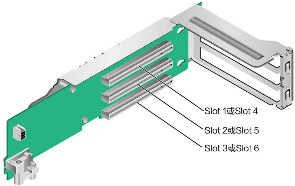
图 6-28 3*x8 Riser 卡
