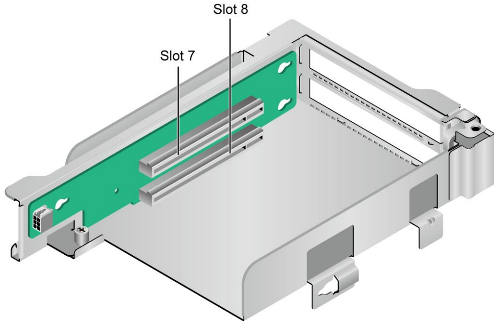
图 6-32 2*x8 Riser 卡
