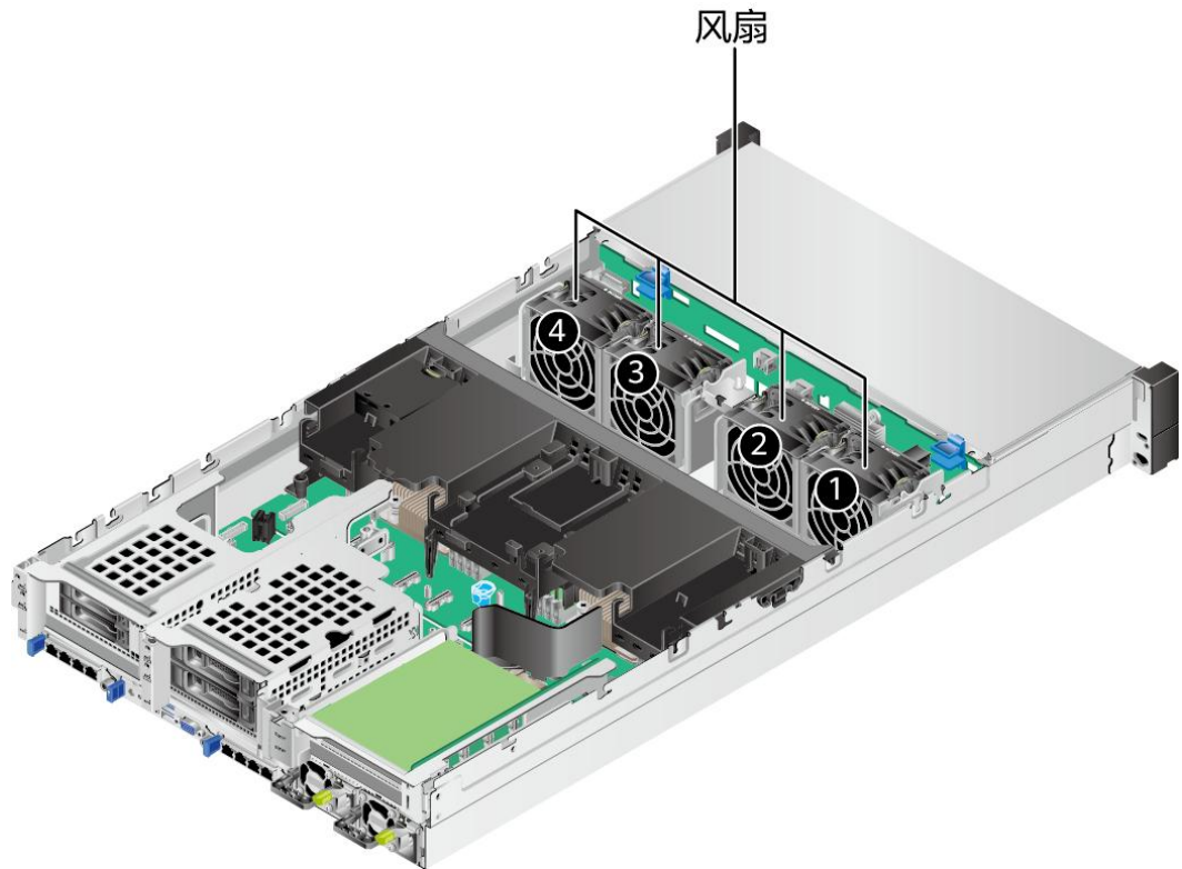
图 6-9 风扇位置图
