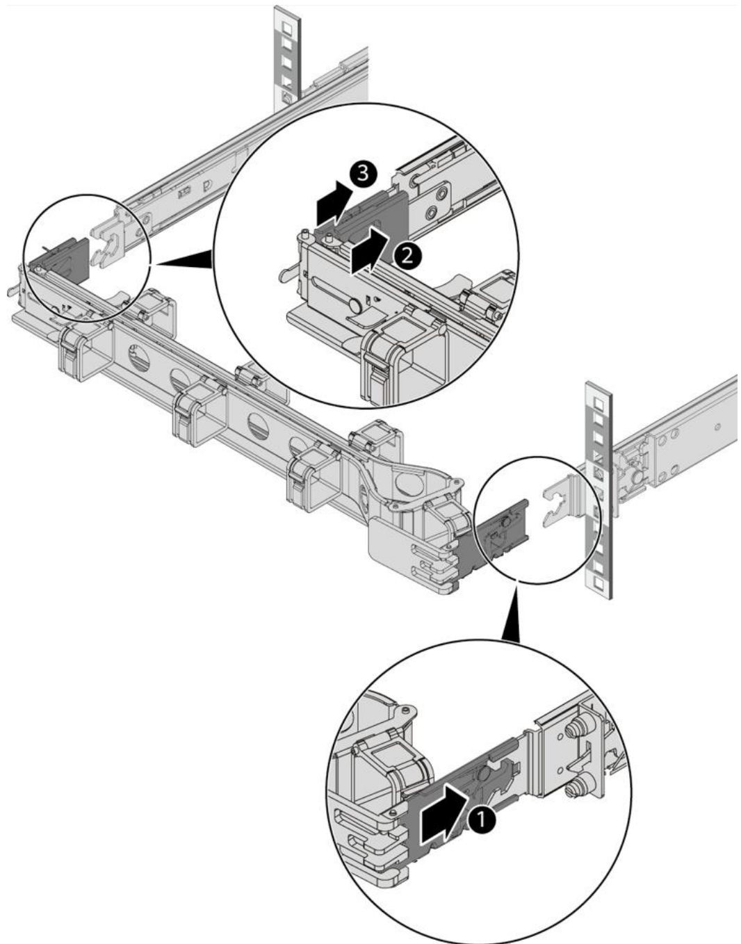
图 9-17 安装理线架
