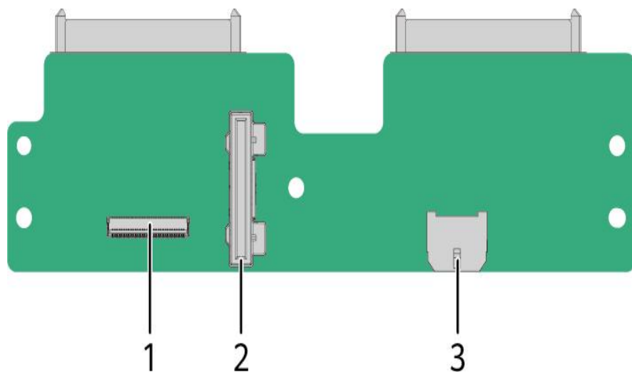
图 5-27 IO 模组 3 水平硬盘背板（上板）
