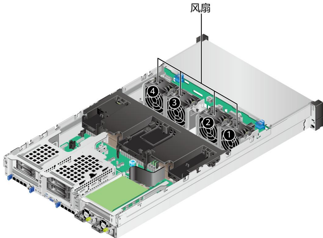
图 5-10 风扇位置图
