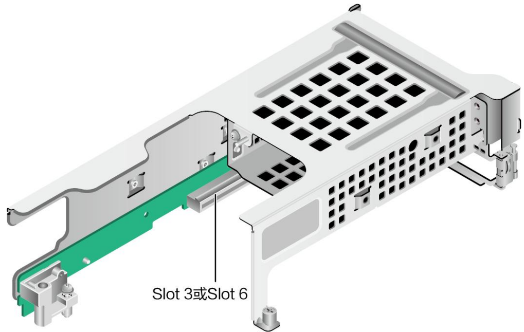
图 5-33 1*x16 Riser 卡
