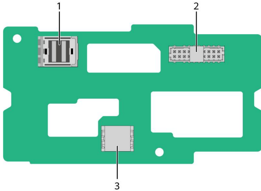
图 5-25 2x3.5 英寸后置硬盘背板
