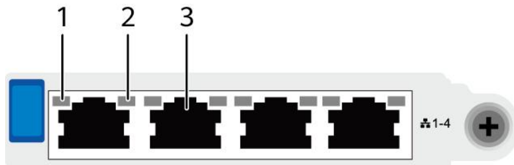
图 5-36 SF221Q (4xGE 电口)
