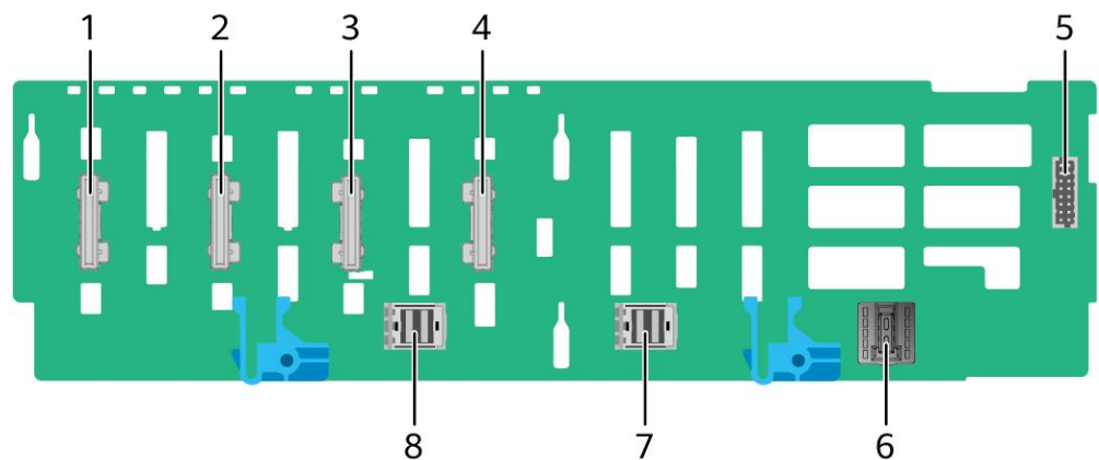
图 5-24 4x2.5 SAS/SATA+8x2.5 NVMe 硬盘配置硬盘背板
