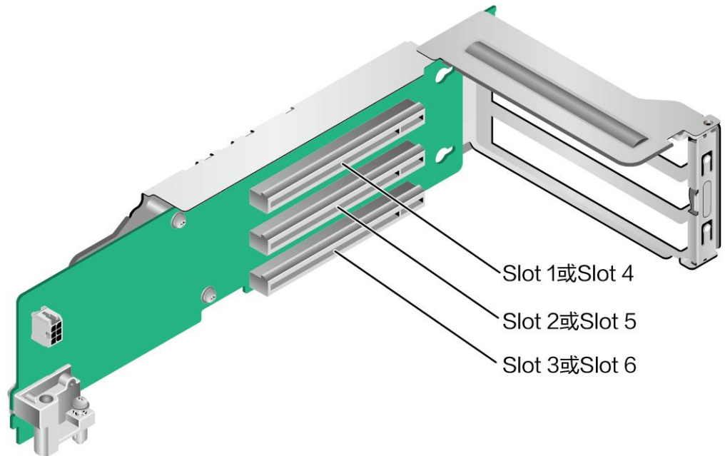
图 5-31 3*x8 Riser 卡
