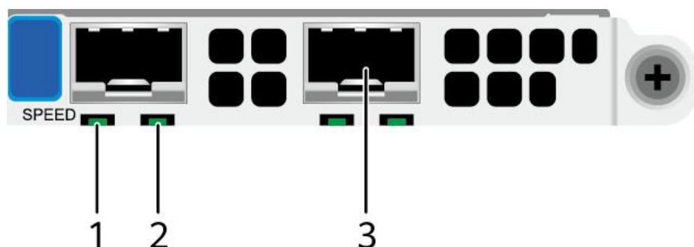
图 5-37 SF223D-H (2x25GE 光口)
