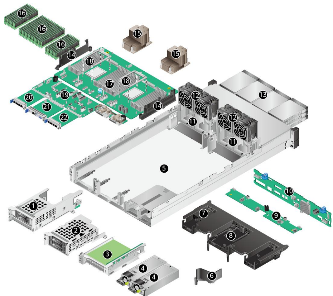
图 3-1 部件
