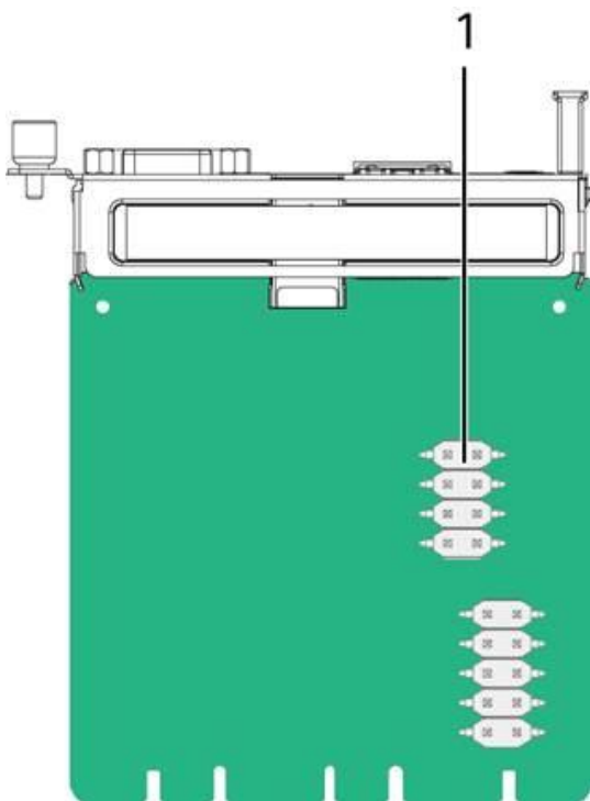
图 5-39 BMC 插卡
