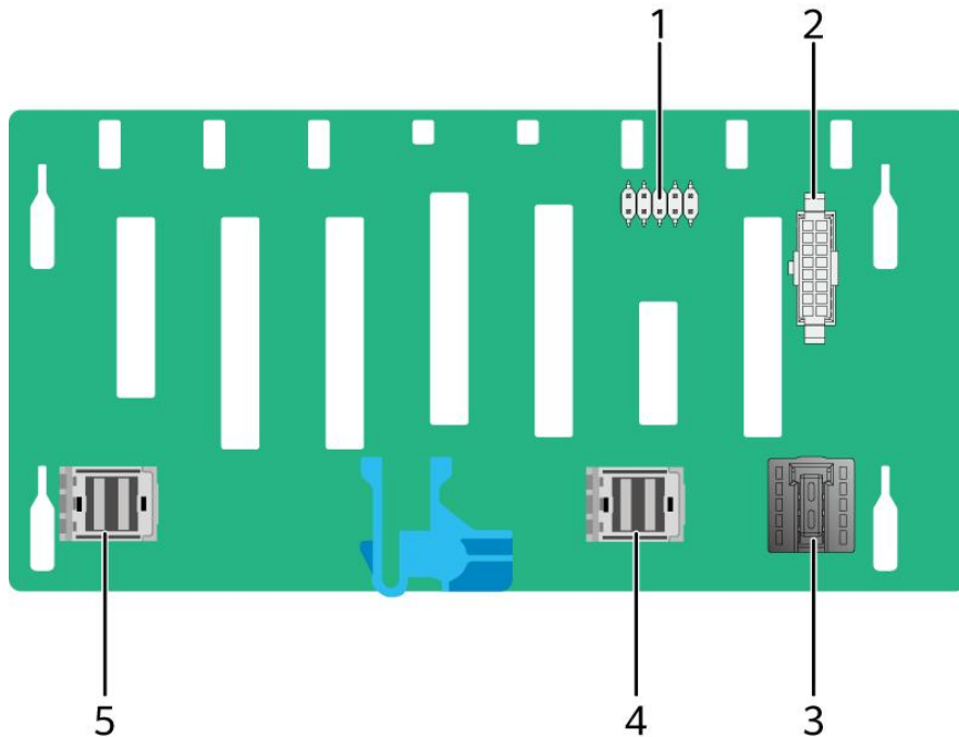
图 5-22 8x2.5 英寸硬盘 RAID 直通配置硬盘背板
