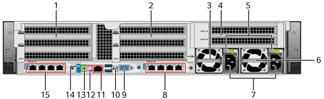
图 5-5 后面板
