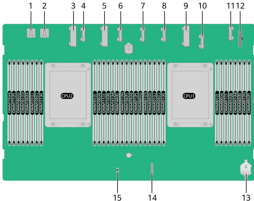
图 5-6 基础板接口
