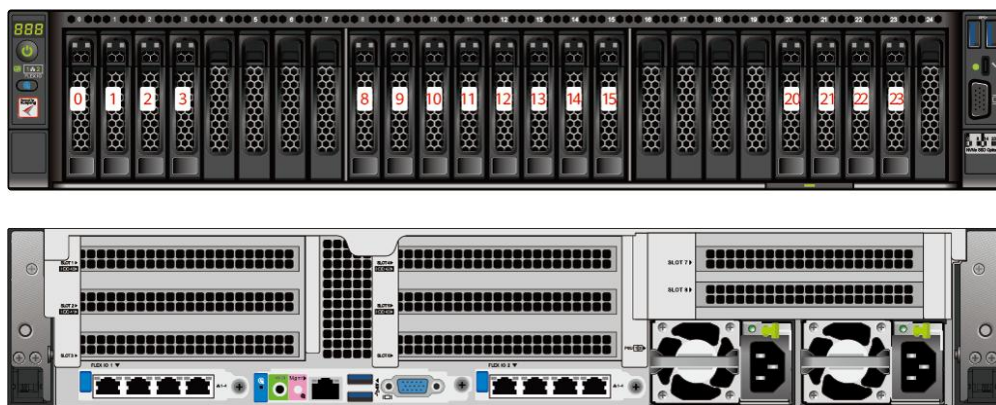
图 5-11 4x2.5 SAS/SATA+12x2.5 NVMe 硬盘配置硬盘编号
