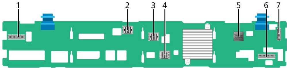
图 5-21 12x3.5 英寸硬盘 EXP 配置硬盘背板
