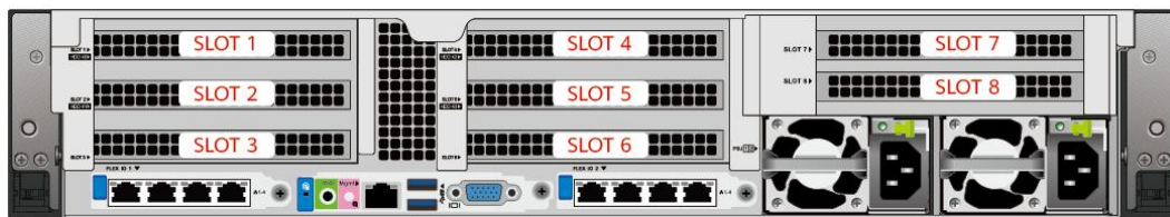
图 5-35 PCIe 插槽
