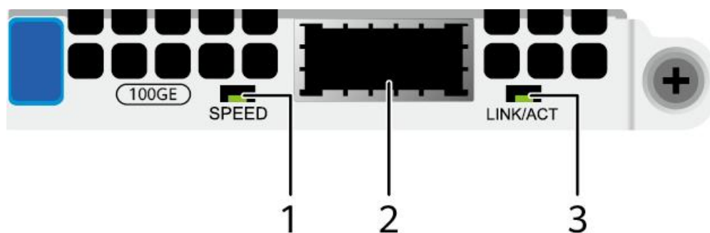
图 5-38 SF225S-H (1x100GE 光口)
