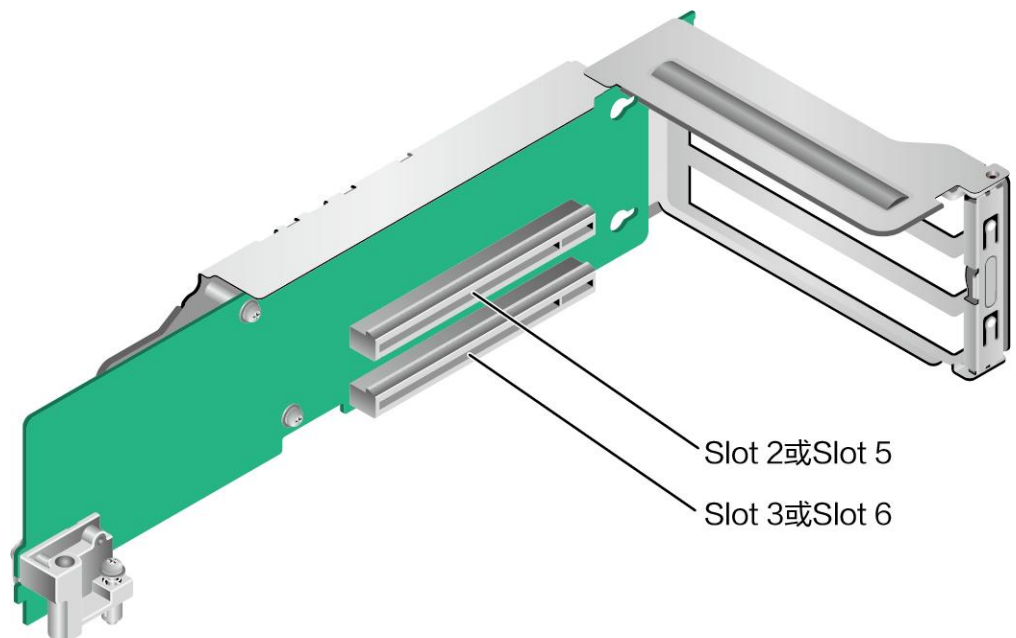
图 5-32 2*x8 Riser 卡
