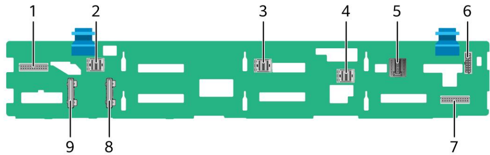
图 5-23 12x3.5 英寸硬盘 RAID 直通配置硬盘背板
