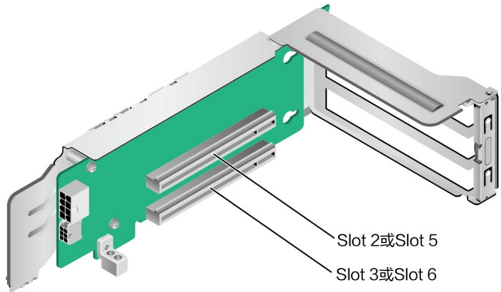
图 5-29 1*x16+ 1*x8 Riser 卡（正面）
