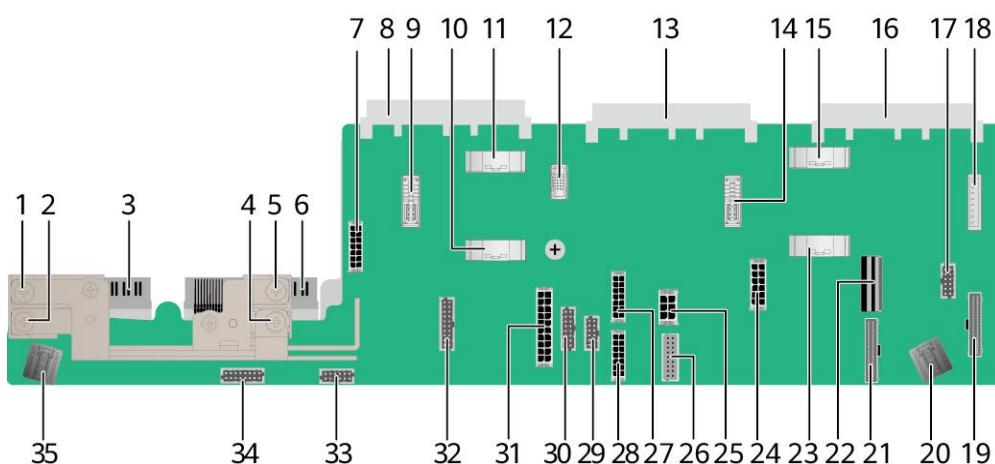
图 5-8 扩展板
