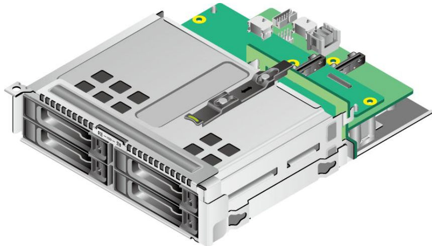
图 5-19 后置 4x2.5 英寸硬盘模组
