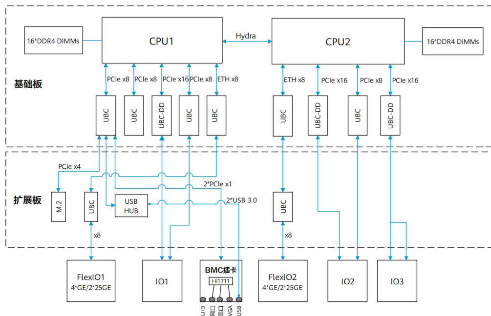
图 4-1 逻辑结构
