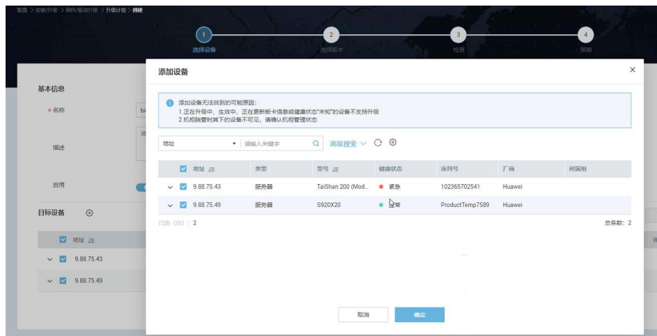
图 2-18 添加设备
