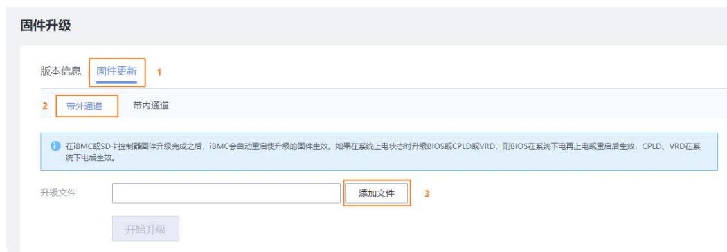
图 2-7 固件更新
