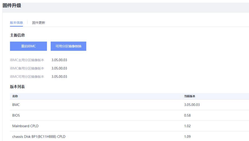
图 2-6 固件升级
