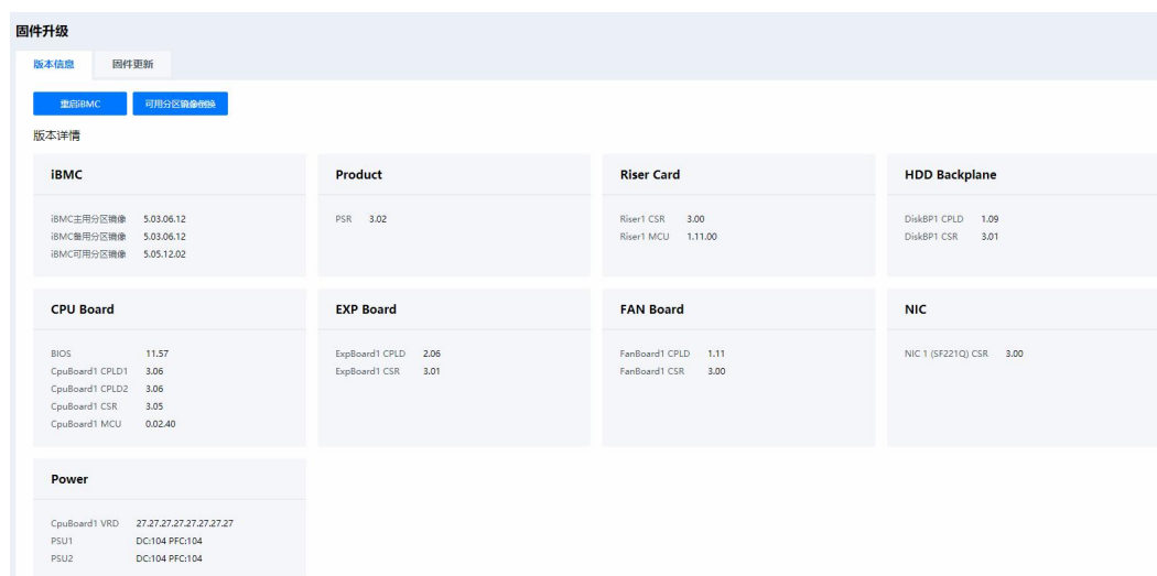
图 2-35 固件升级
