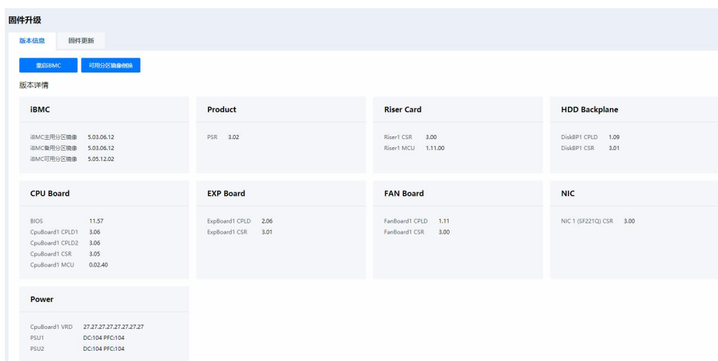
图 2-31 固件升级
